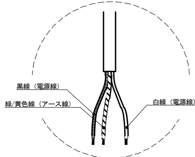
電源ケーブル先端部拡大
